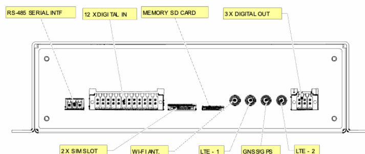
IoT Box EVO: vista posteriore
