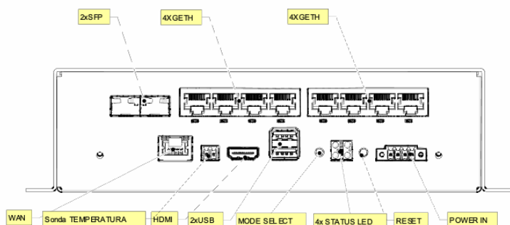
IoT Box EVO: vista anteriore
